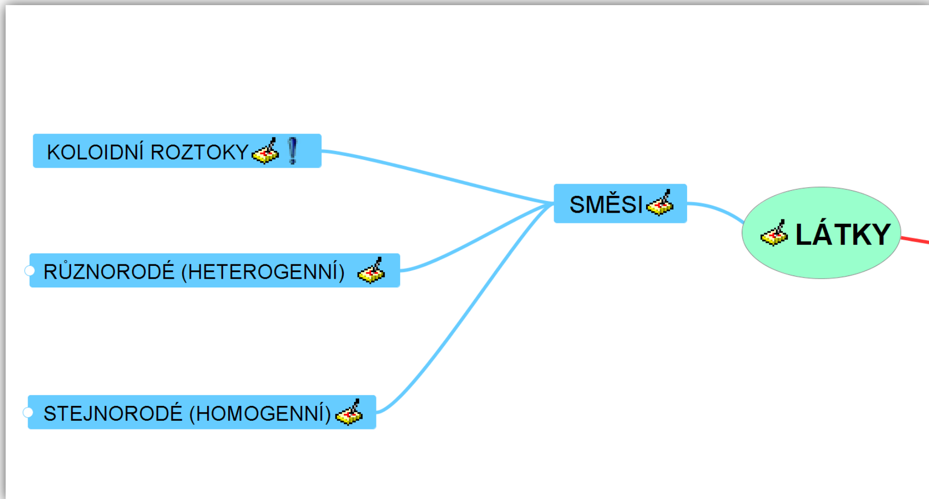
Obrázek č. 3: Rozdělení směsí.
