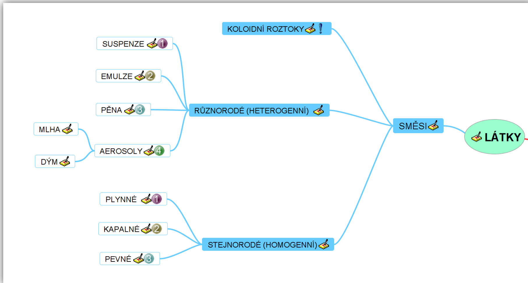
Obrázek č. 5: Rozdělení různorodých a stejnorodých směsí.
