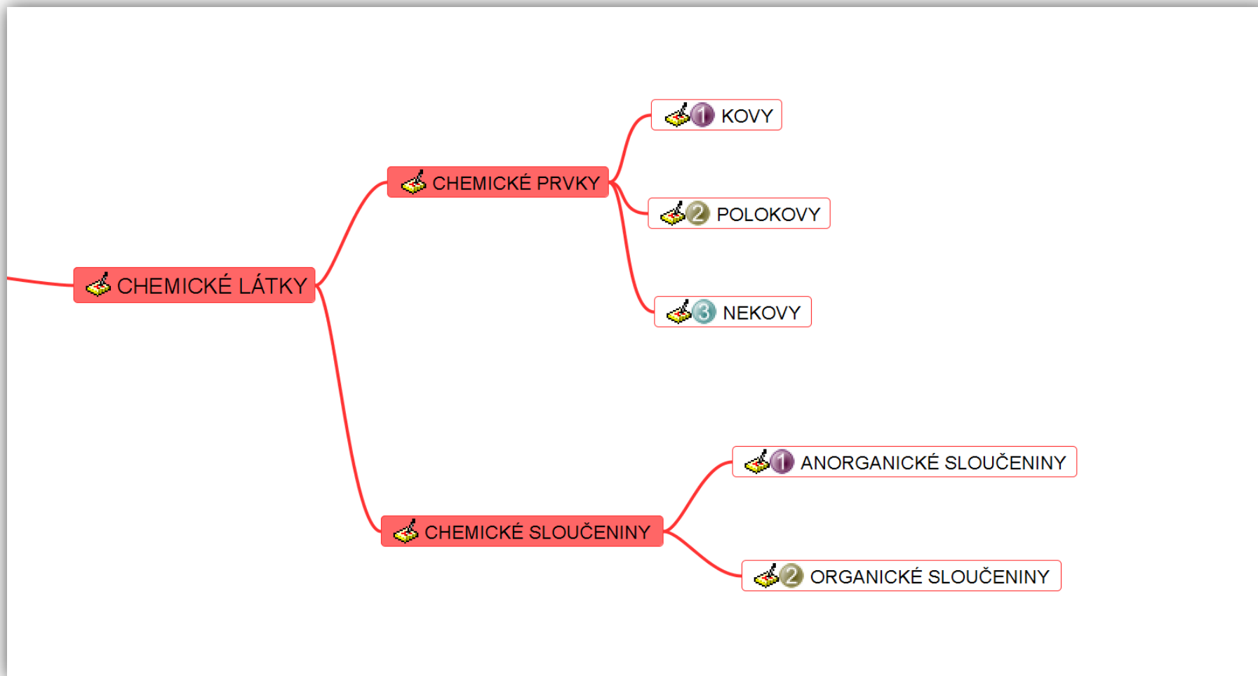
Obrázek č. 4: Rozdělení chemických prvků a chemických sloučenin.
