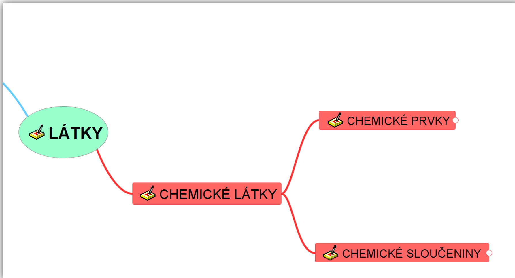
Obrázek 2: Rozdělení chemických látek.
