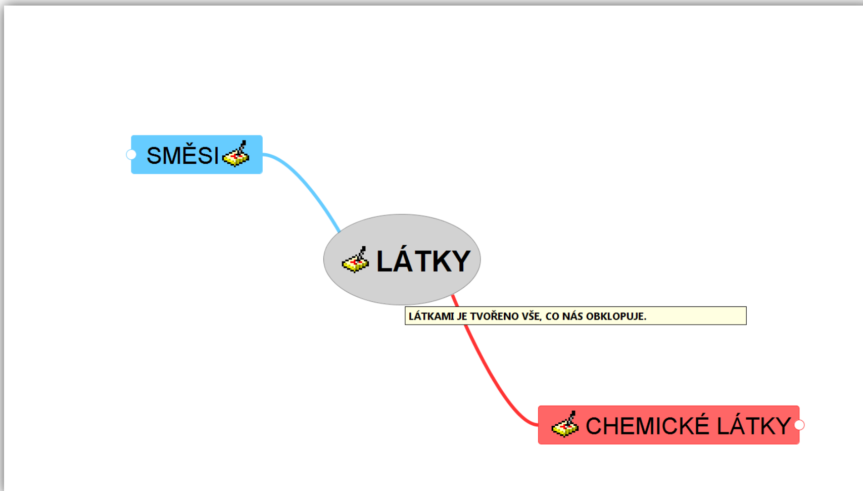
Obrázek 1: Základní rozdělení látek. U pojmu látky je vložena poznámka, kterou dle potřeby můžeme skrýt.
