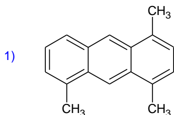
1,4,5-trimethylantracén
