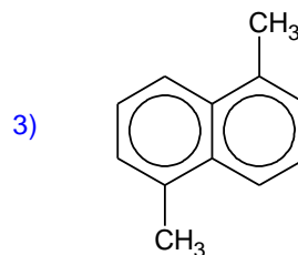
1,5 - dimethylnaftalen
