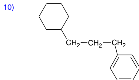
1-fenyl-3-cyklohexylpropan (3-cyklohexylpropyl)benzen
