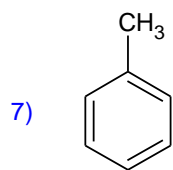
toluen methylbenzen
